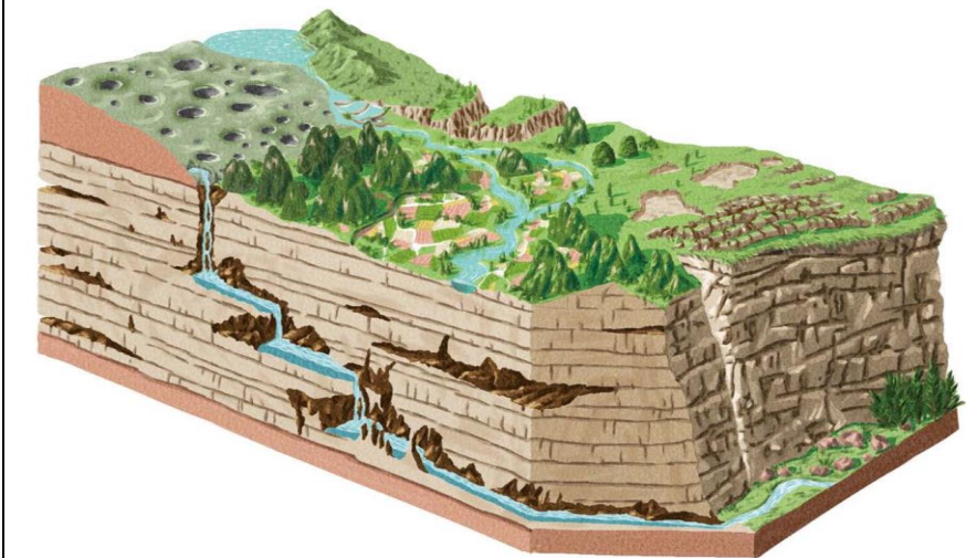
石灰岩
